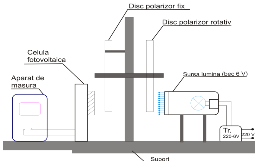
Figura 4. Dispozitivul experimental
